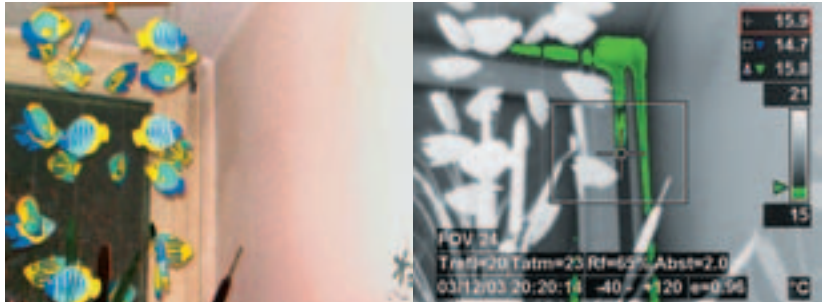
Imágen visual e infrarroja de un dormitorio. La imagen infrarroja nos muestra claramente las zonas delicadas en donde el moho puede crearse.
