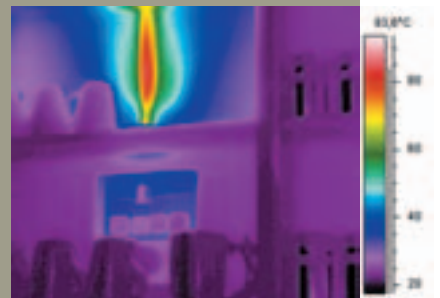
Calentador de gas construido muy cerca de la pared constituye un riesgo de incendio
