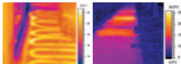
Calefacción suelo radiante
