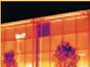
Ventanas de panel sencillo entre ventanas con paneles dobles
