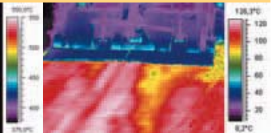
Distribución de temperaturas en pavimentos asfaltados
