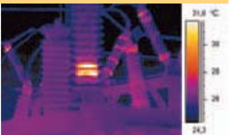
Defectos en aislantes
