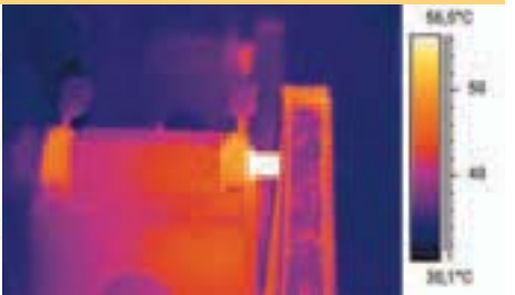
Cojinetes calientes
